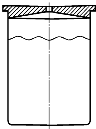
Рисунок 1 — Металлический пикнометр
